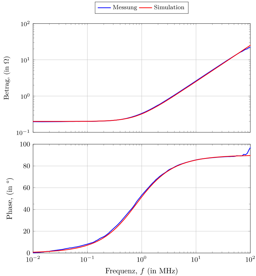
Abbildung 3.38: Impedanzmessung und Simulation einer Batteriezelle
