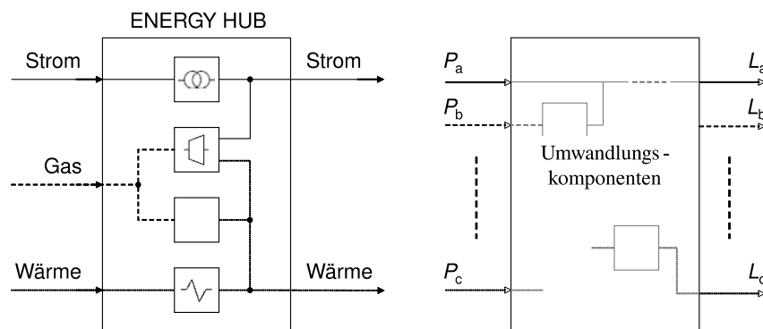
Abbildung 3.16: Schematische Darstellung eines Energy Hub
