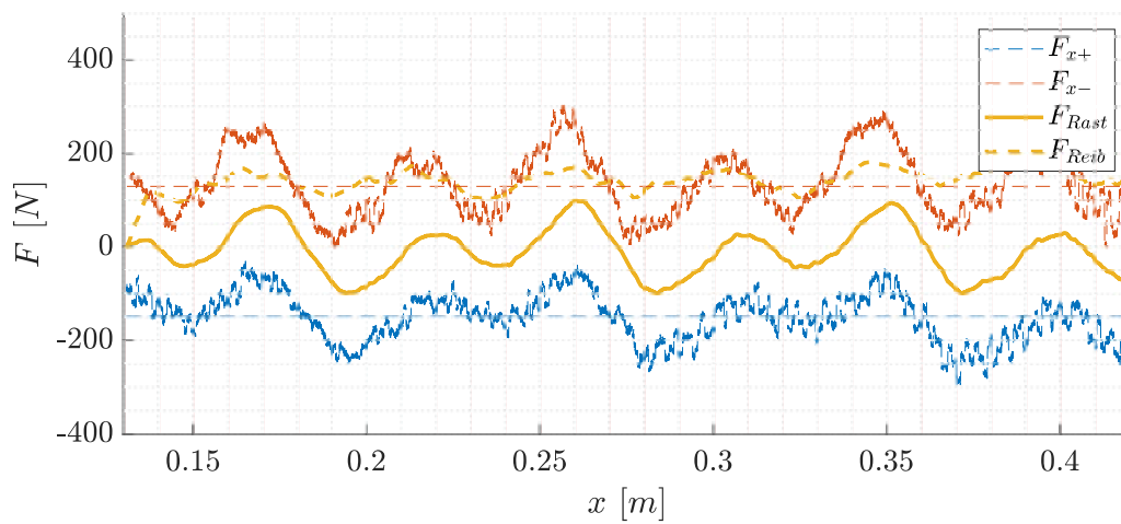
Abbildung 3.14: Gemessener Rastkraftverlauf des Labormusters
