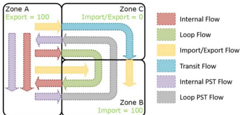
Abbildung 3.18: ENTSO-E Lastflussdefinitionen erweitert um PST-Flüsse
