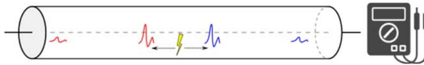
Abbildung 3.24: Schematische Signalübertragung einer Teilentladung auf einem Energiekabel zwischen Ort der Entstehung und der nächsten möglichen Messstelle
