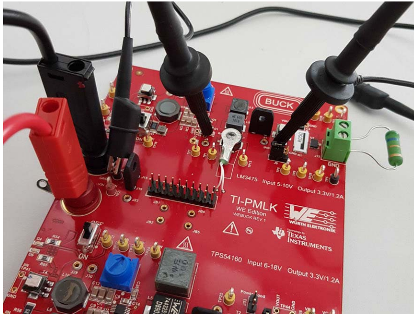
Abbildung 2.5: Im Sommersemester 2020 führten Studierende in der Lehrveranstaltung „EMV-Messtechnik“ in Eigenregie verschiedene Experimente mit dem Tiefsetzsteller-Board TI-PMLK BUCK von Würth Elektronik bzw. Texas Instruments durch.
