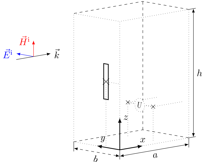
Abbildung 3.34: Geometrie einer geschlitzten, quaderförmigen Apertur. Im Inneren befindet sich ein elektrisch großer Dipol. Die Anregung wird entweder durch ein äußeres, einfallendes Feld oder eine Spannungsquelle am Dipol realisiert.
