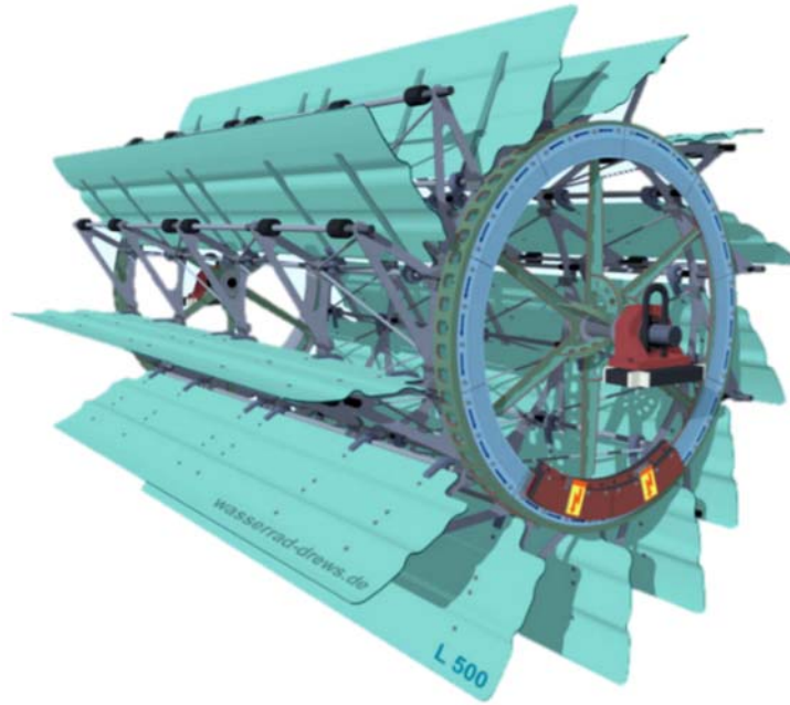
Abbildung 3.10: Drew'sches Klappschaufelwasserrad mit integriertem Ringsegmentgenerator
