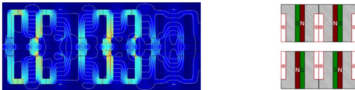
Abbildung 3.12: Finite-Elemente-Simulationsmodell der flussgeschalteten permanentmagnetischen Synchronmaschine mit Wicklungsverschaltung und Magnetanordnung
