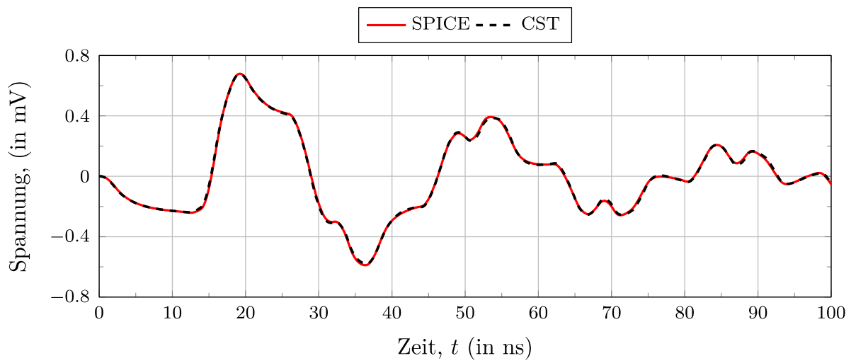
Abbildung 3.36: Simulationsergebnisse der geschirmten Leitung
