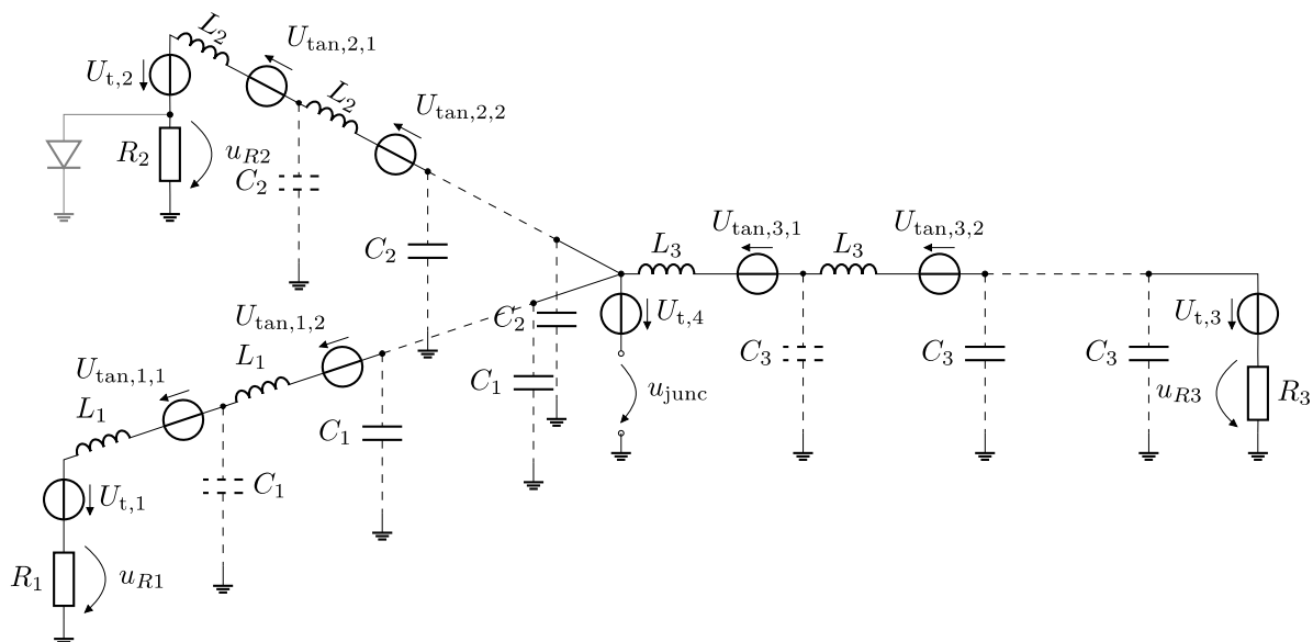
Abbildung 3.41: Ersatzschaltbild eines beispielhaften, nichtlinear-abgeschlossenen Leitungsnetzwerks aus drei Leitungen mit einem gemeinsamen Knotenpunkt
