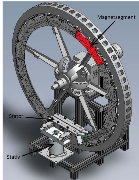
Abbildung 3.11: Versuchsstand mit Ringsegmentgenerator
