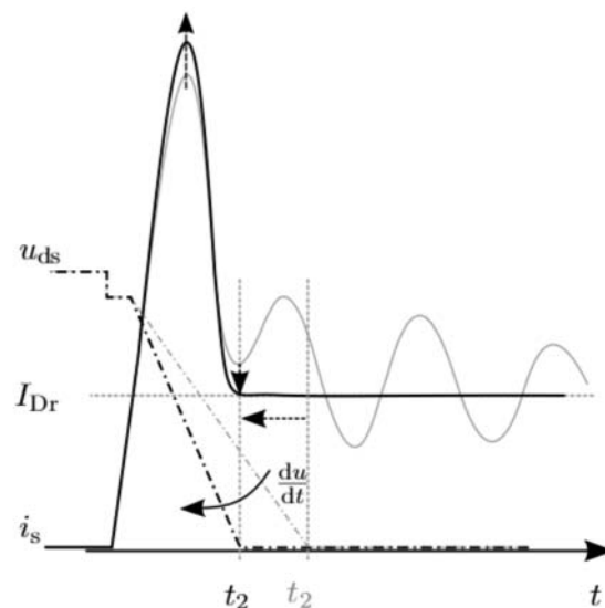
Abbildung 3.55: Einstellen der Spannungsflanke, um Stromoszillation zu minimieren
