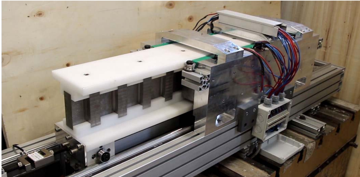
Abbildung 3.13: Labormuster zur Verifikation der Simulationsergebnisse und Erbringung des Funktionsnachweises
