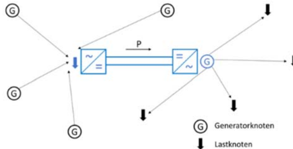
Abbildung 3.19: Prinzip der HVDC Flows mit gleichmäßig proportionaler Aufteilung
