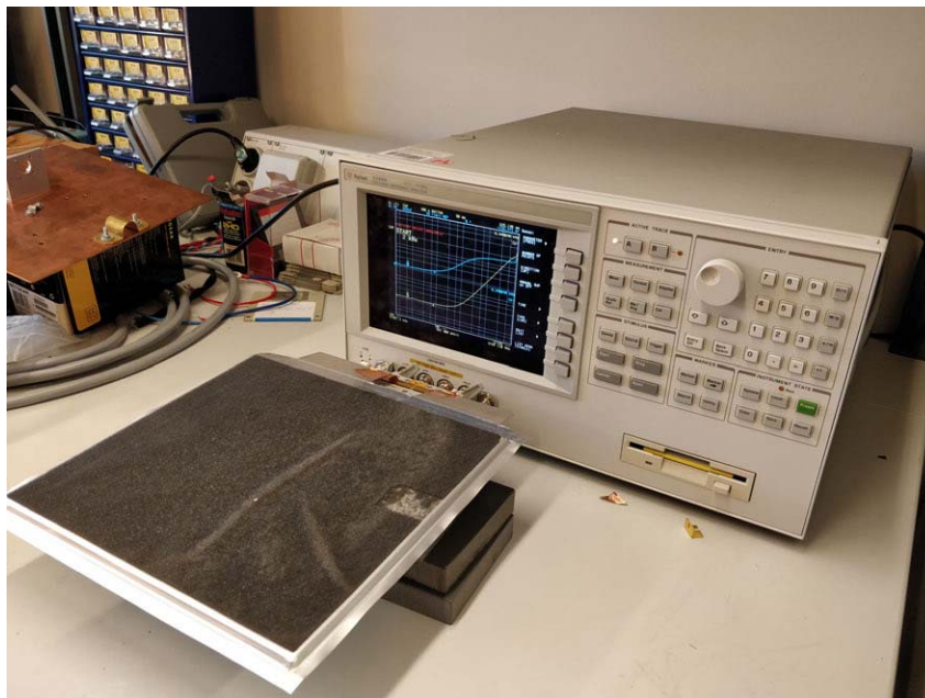
Abbildung 3.37: Messaufbau einer Batteriezelle
