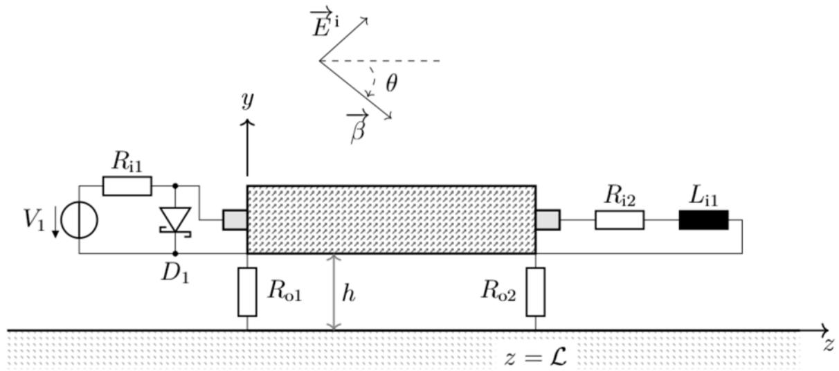
Abbildung 3.35: Simulationsbeispiel der geschirmten Leitung.
