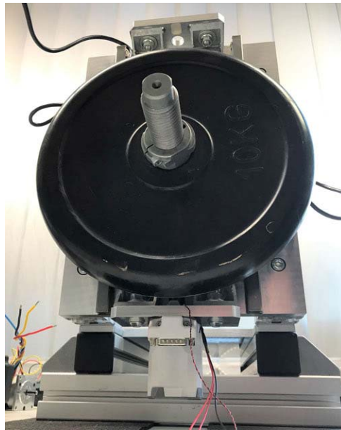
Abbildung 3.8: Belastungsstand. Der unten angeflanschte SMELA-Aktuator hebt je nach Leistungsklasse bis zu 30 kg, 65 kg oder 80 kg.
