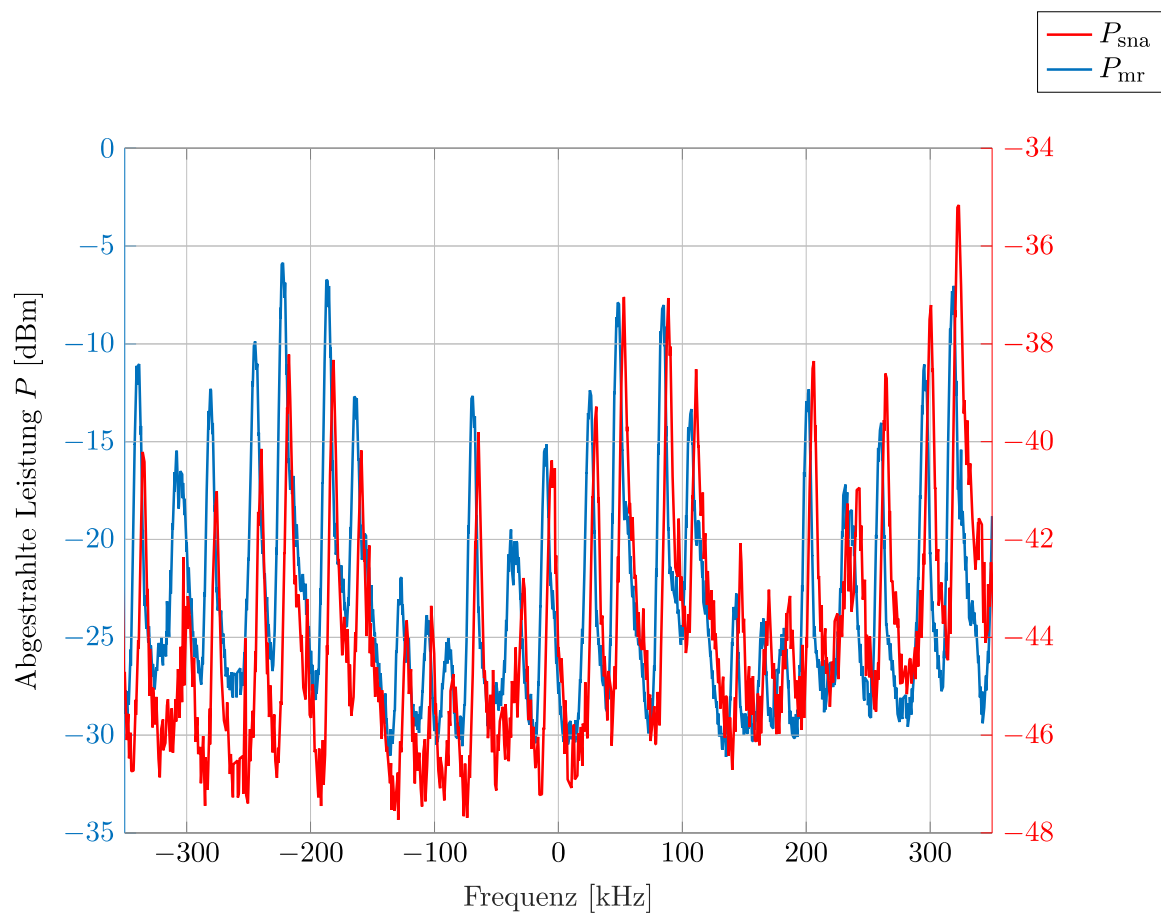
(b) Leistungsspektrum-Vergleich des Testsetups mit dem MRT
