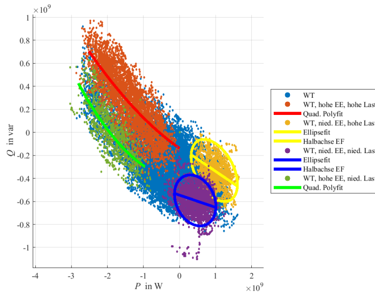
Abbildung 3.21: Wirk- und Blindleistungsflüsse eines Umspannwerks im Jahr 2018
