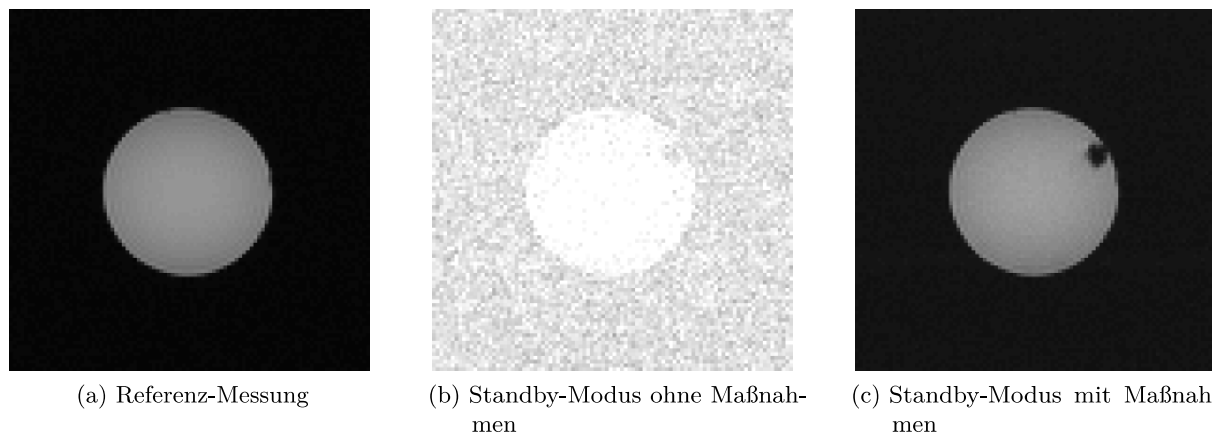
Abbildung 3.33: MRT-Bilder der Referenz-Messung sowie der Messung mit und ohne Entstör-Maßnahmen im Standby-Modus des Mikrowellenablationsgenerators
