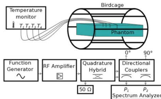
(a) Schematischer Messaufbau
