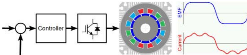
Abbildung 3.2: Regelung von Maschinen nicht sinusförmiger elektromotorischer Kraft
