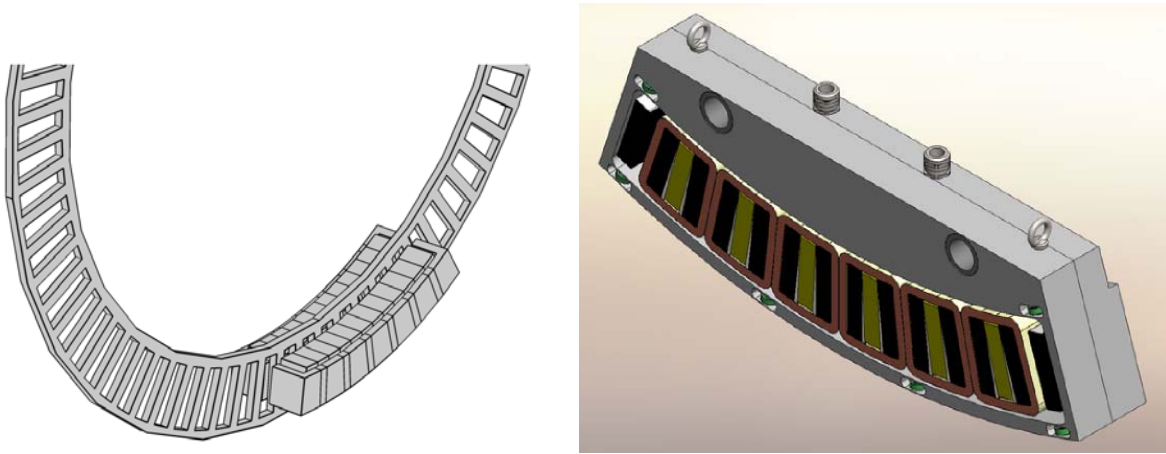
Abbildung 3.15: Konstruktionszeichnungen des Prinzips Ringsegmentgenerator (links) und einer Statorhälfte des Prototypen (rechts)
