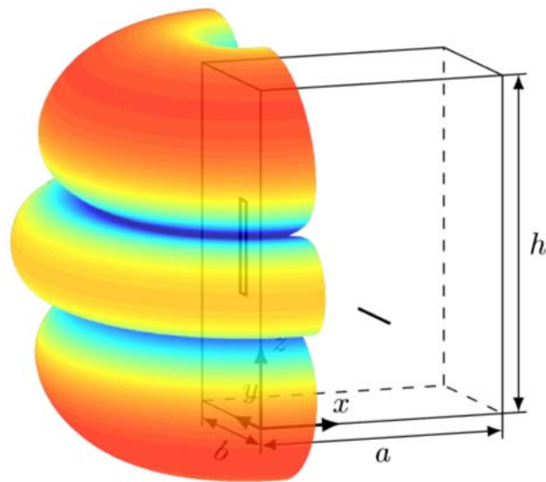
Abbildung 3.46: Abstrahlung eines elektrisch langen Schlitzes in einem quaderförmigen Hohlraumresonator
