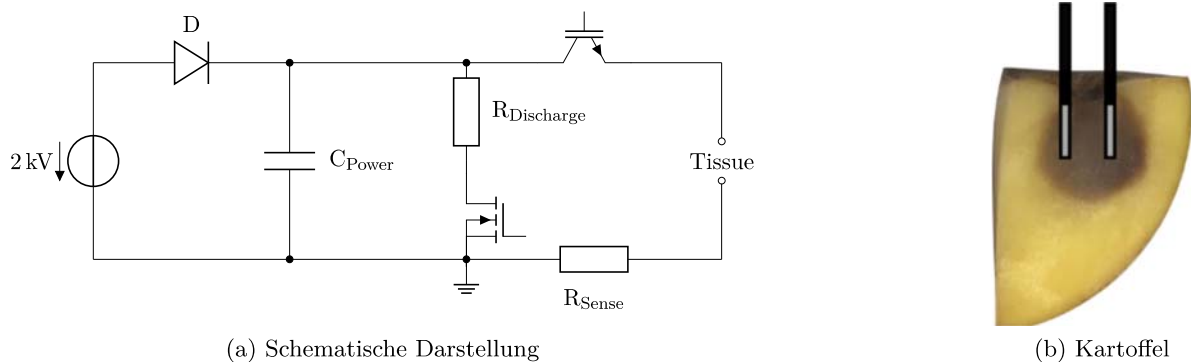
Abbildung 3.29: Schematische Darstellung des IRE-Geräts und Resultat der IRE in einer Kartoffel
