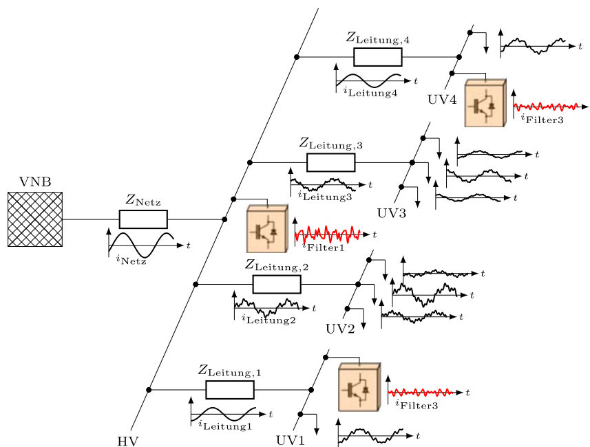
Abbildung 3.43: Prinzipdarstellung verteilter OberschwingungsfILTER
