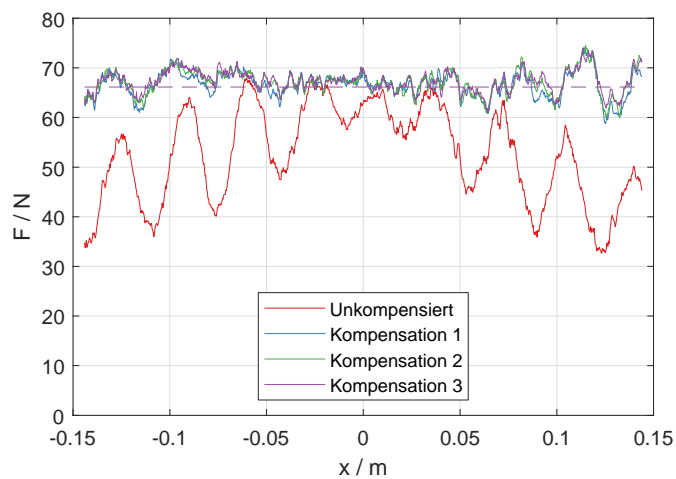
(a) Vergleich der Maschinenkraft mit und ohne Kompensation
